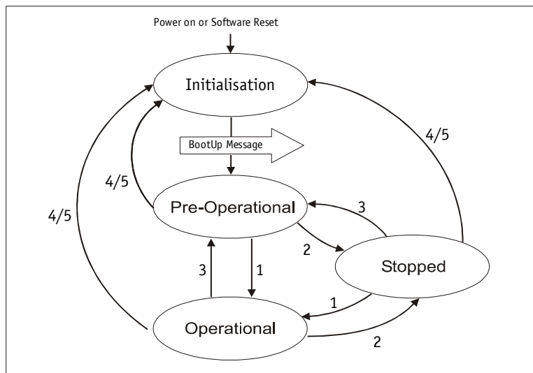
Fig. 9: State Diagramm
