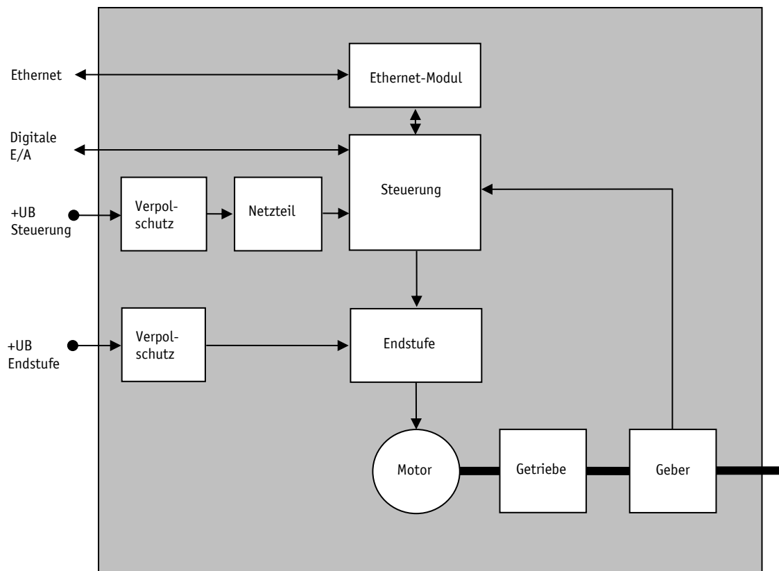
Abb. 22: Blockschaltbild
