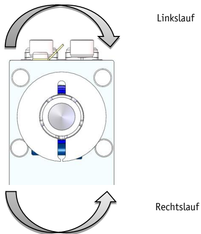
Abb. 13: Drehrichtung
