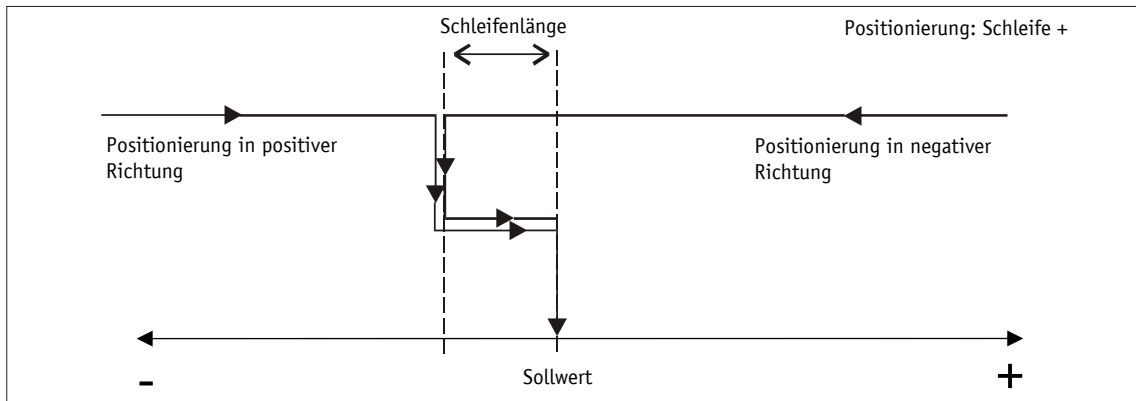
Abb. 8: Positionierung Schleife+
