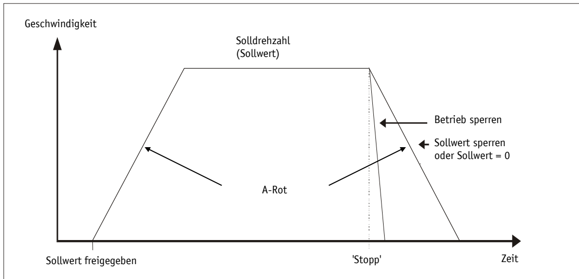
Abb. 14: Rampe Drehzahlmodus
