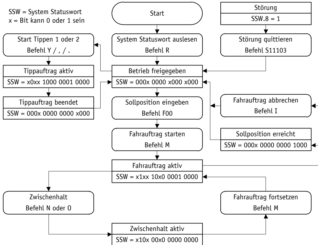
Abb. 18: Ablaufplan Positioniermodus Serviceprotokoll
