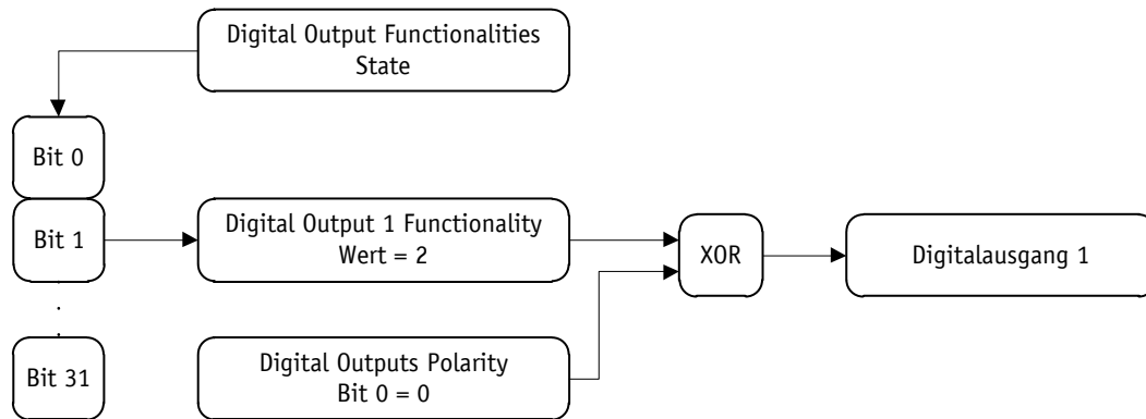
Abb. 11: Beispielkonfiguration Digitalausgang
