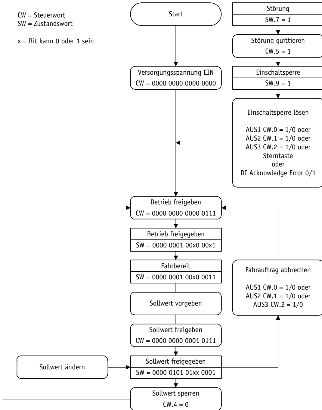
Abb. 15: Ablaufplan Drehzahlmodus
