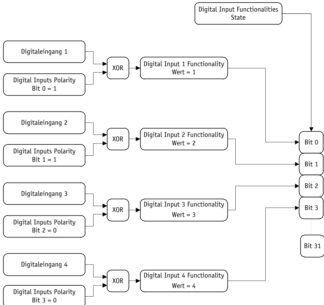
Abb. 10: Beispielkonfiguration Digitaleingänge
