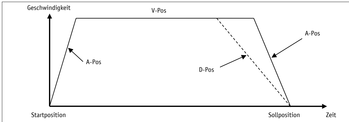
Abb. 4: Rampenfahrt Positioniermodus direkt
