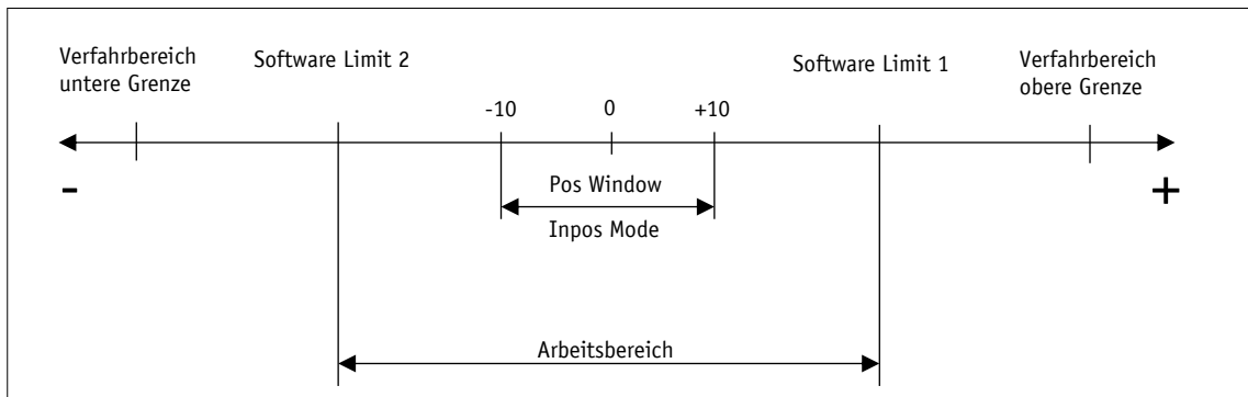
Abb. 5: Positioniermodus
