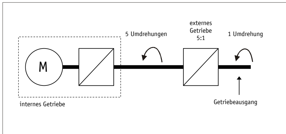
Abb. 3: externes Getriebe
