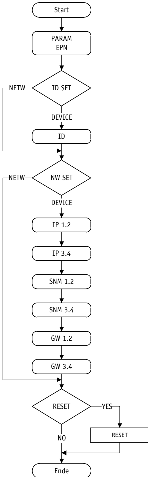
Abb. 16: Einstellung des Stationsnamens und der IP-Konfiguration
