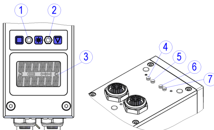
Abb. 1: Anzeigen und Bedienelemente
