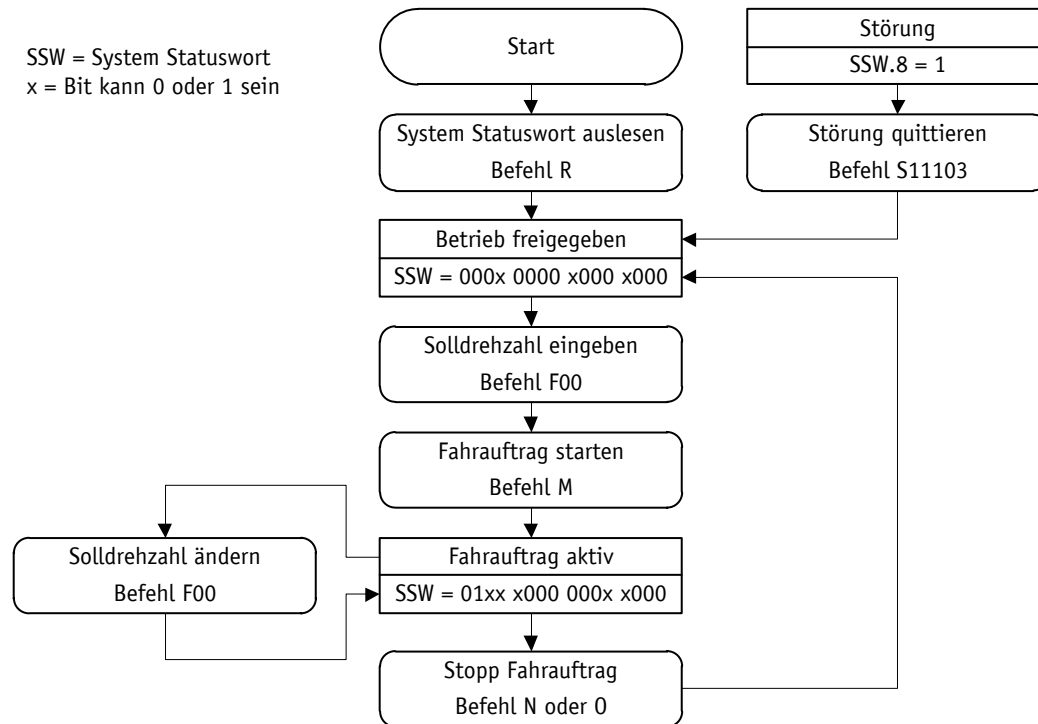
Abb. 19: Ablaufplan Drehzahlmodus Serviceprotokoll
