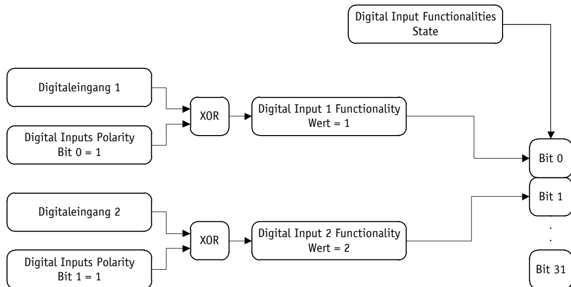
Abb. 6: Beispielkonfiguration Endschalter
