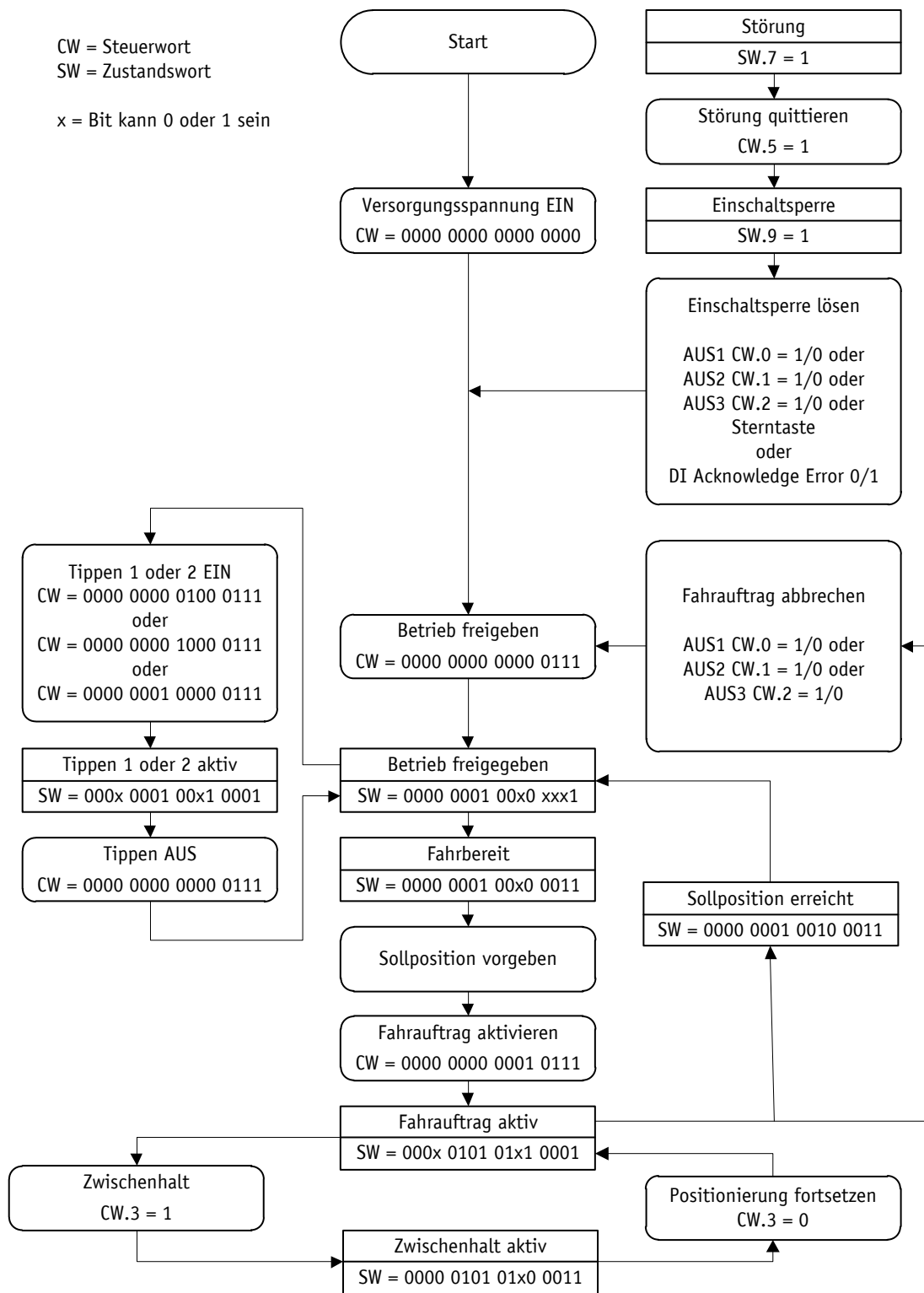
Abb. 9: Ablaufplan Positioniermodus
