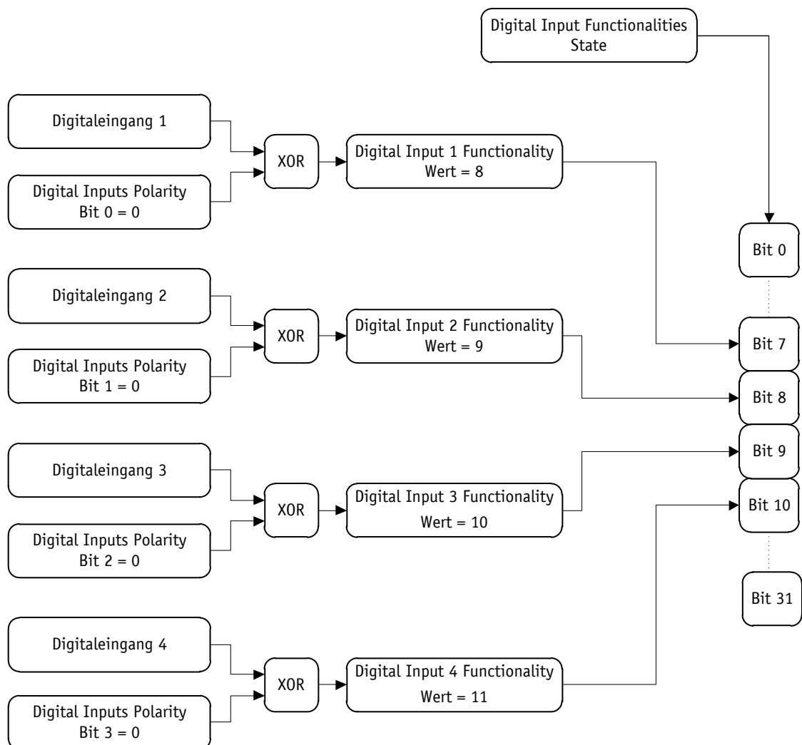
Abb. 12: Beispielkonfiguration der Digitaleingänge für den PCM
