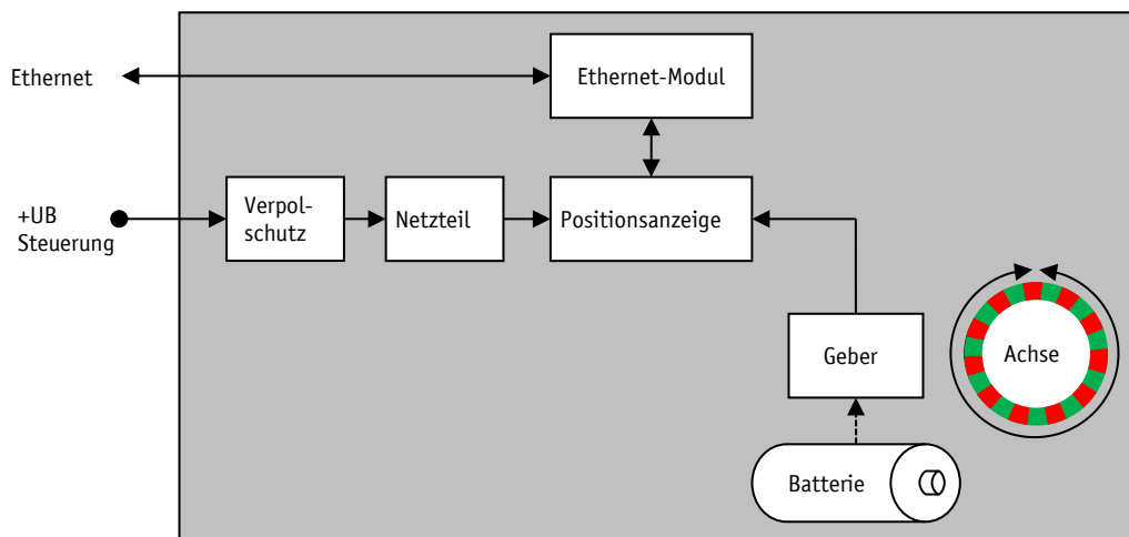
Abb. 8: Blockschaltbild
